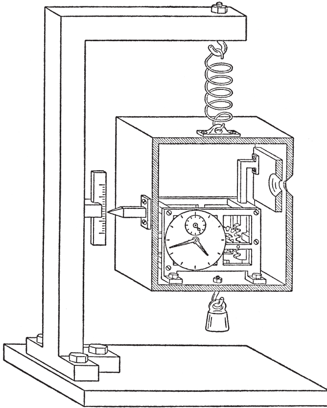
Abb. 4: Einsteins Kasten mit Uhr und Feder
